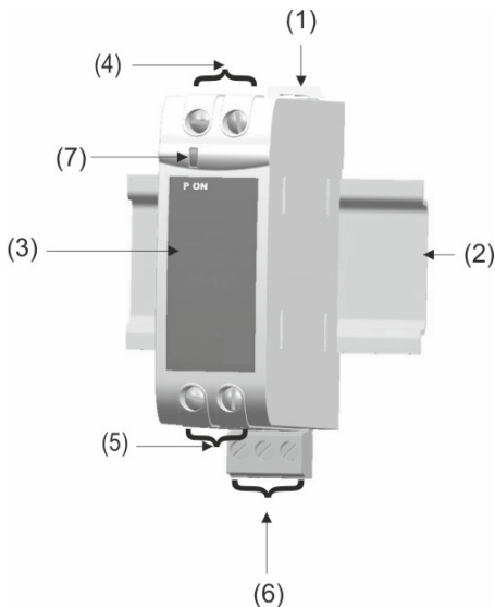
Rys. 1: Przegląd elementów przetwornika
