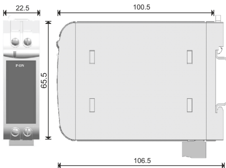
Rys. 7. Wymiary przetwornika.
