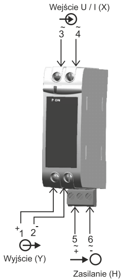
Rys. 6. Widok z przodu wraz ze schematem podłączeń zewnętrznych.
